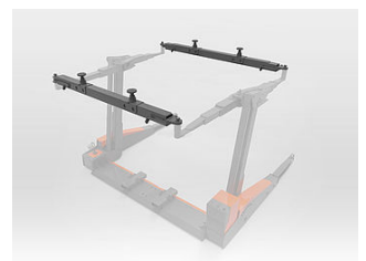
FHB3500-Z-TR03 2 Traversen, 3,5 t, Länge 2826 mm / 2566 mm
