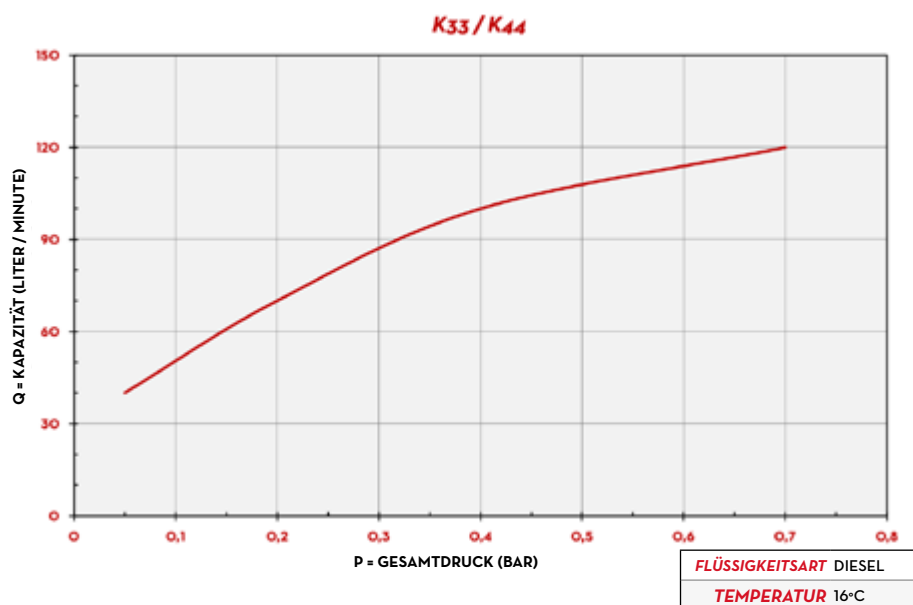
TAUMELSCHIEBENSYSTEM
