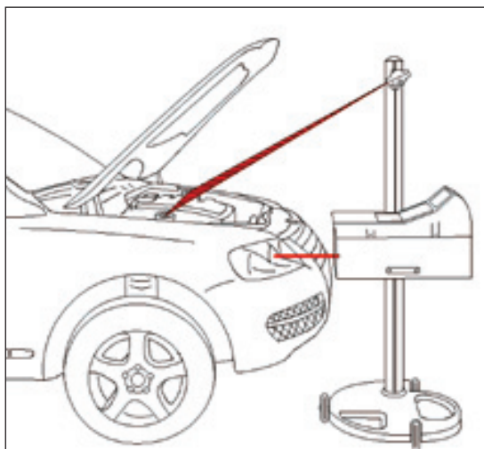
Höheneinstellung mittels Laser
